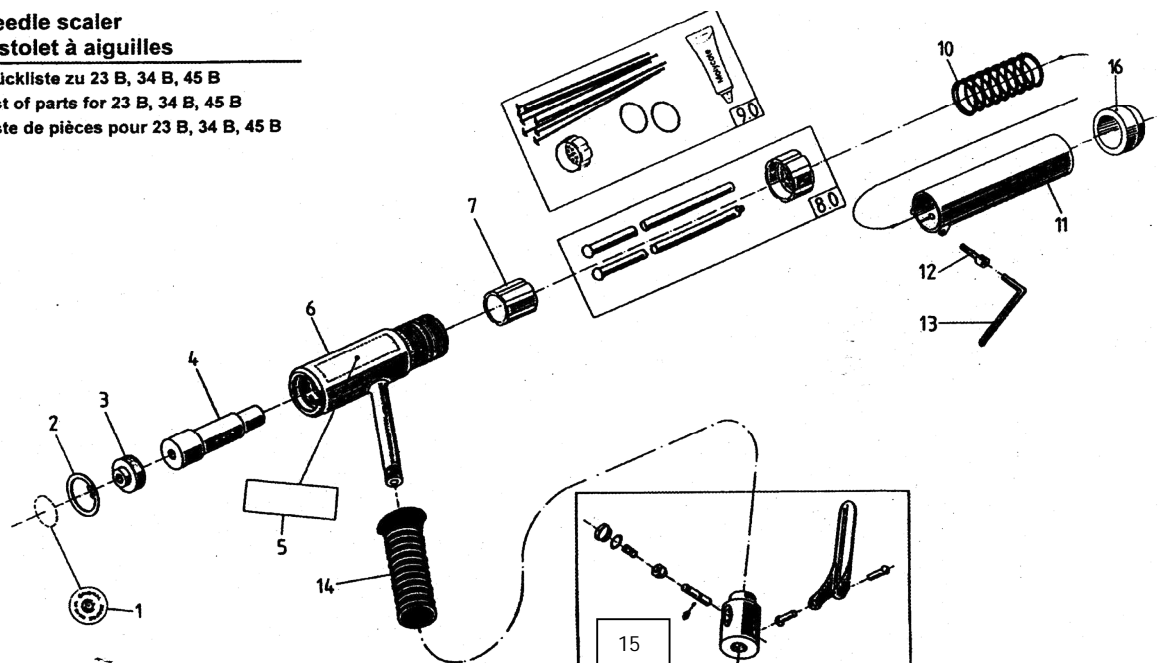
Onderdelenlijst Naaldenbikhamer
